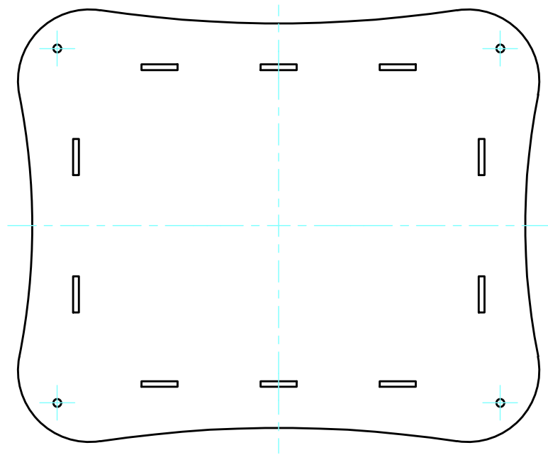
下カバー裏面 / Bottom cover Backside
